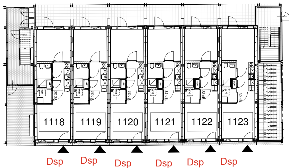
MAKERSKADE blok 5 begane grond
