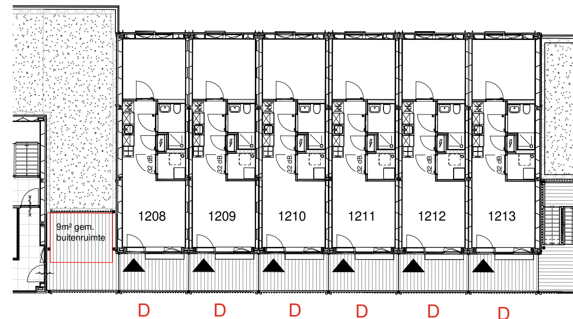
blok 6c eerste verdieping
