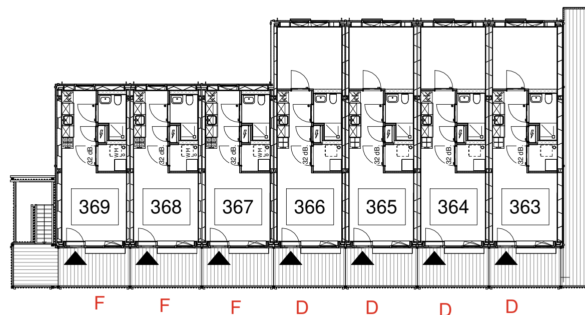
blok 4a derde verdieping
