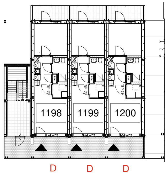
blok 6a begane grond
