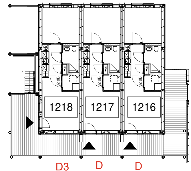
blok 6a tweede verdieping
