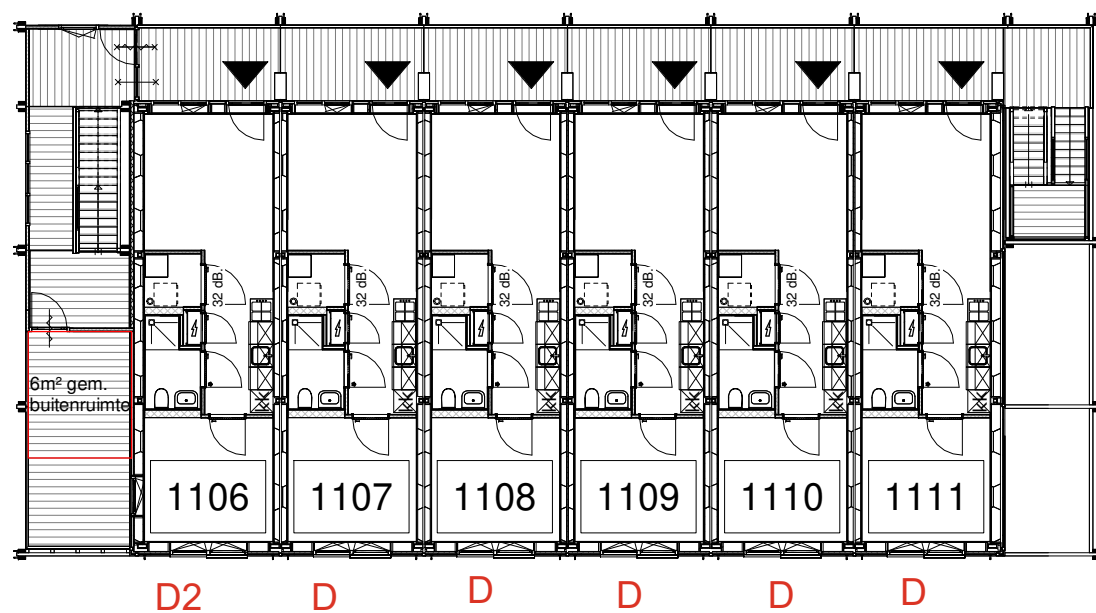
blok 5 tweede verdieping
