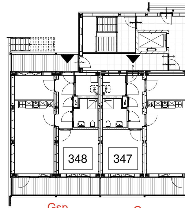
Gsp G blok 4b tweede verdieping
