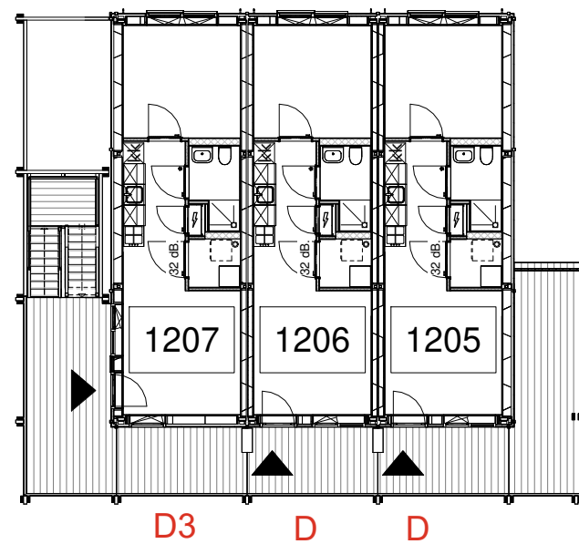
blok 6a eerste verdieping
