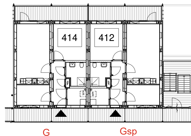
blok 4d tweede verdieping
