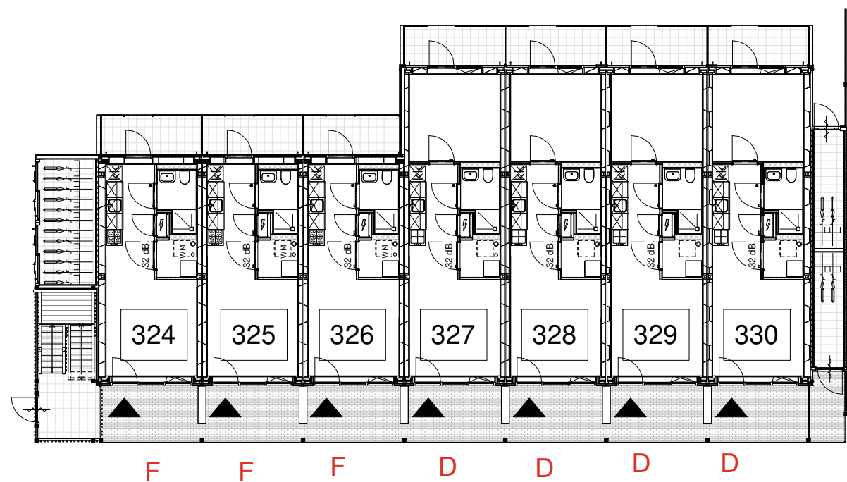
blok 4a begane grond
