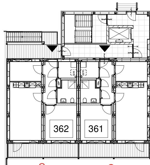
Gsp G blok 4b derde verdieping
