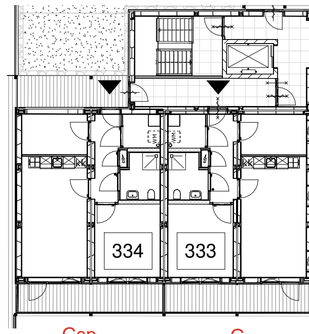
Gsp G blok 4b eerste verdieping
