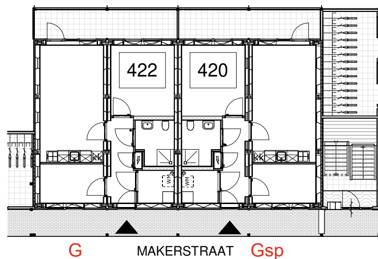
blok 4d begane grond
