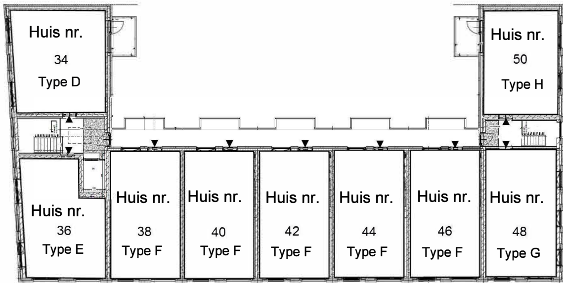
2e verdieping
