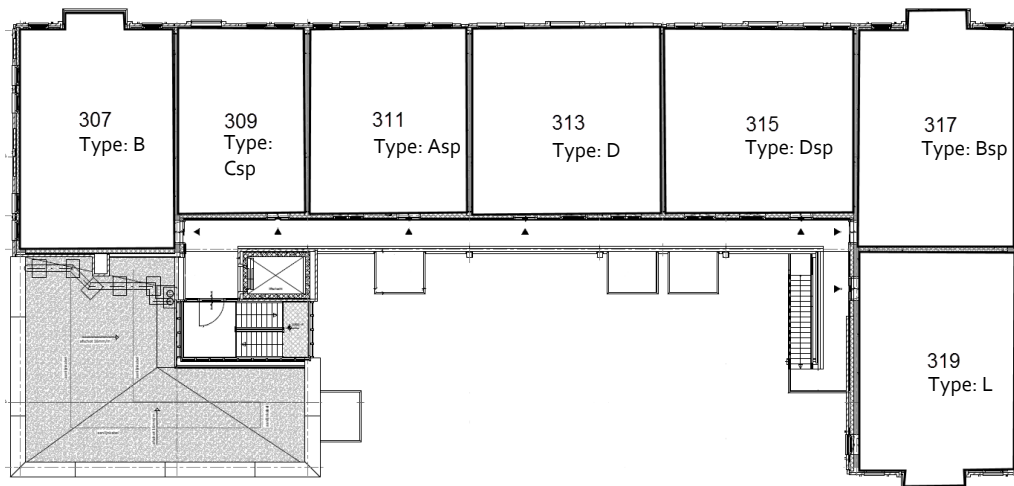
4e verdieping blok 5G
